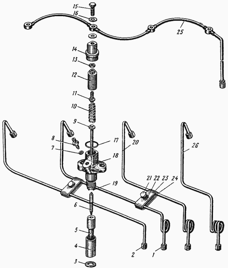
Рис. 12. Форсунки и топливопроводы
